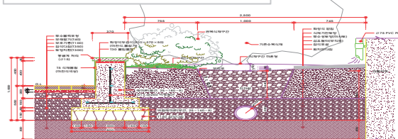
▲ 침투통 및 침투형 빗물받이 단면도
