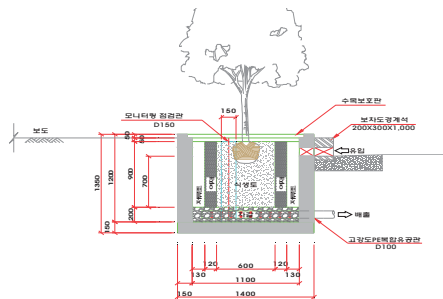
▲ 트리필터박스 단면도
