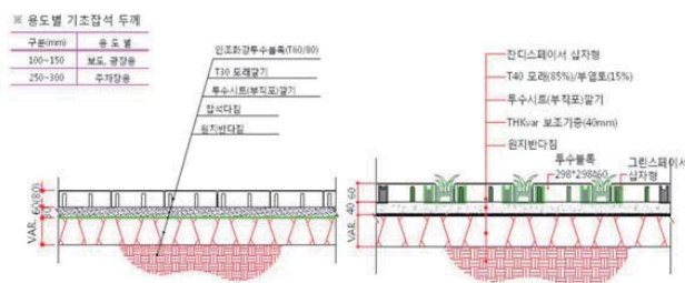
▲ 보도용 투수포장 단면 상세도
