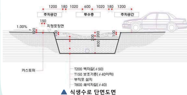
▲ 식생수로 단면도면
