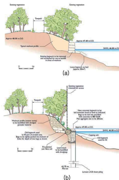
템즈강 하안 침식 방지 공법
