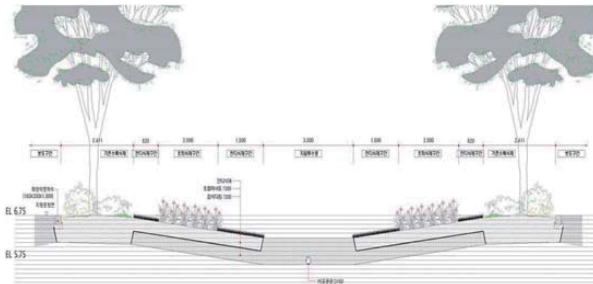
▲ 침투도랑 단면 상세도
