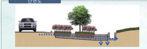
단면도
